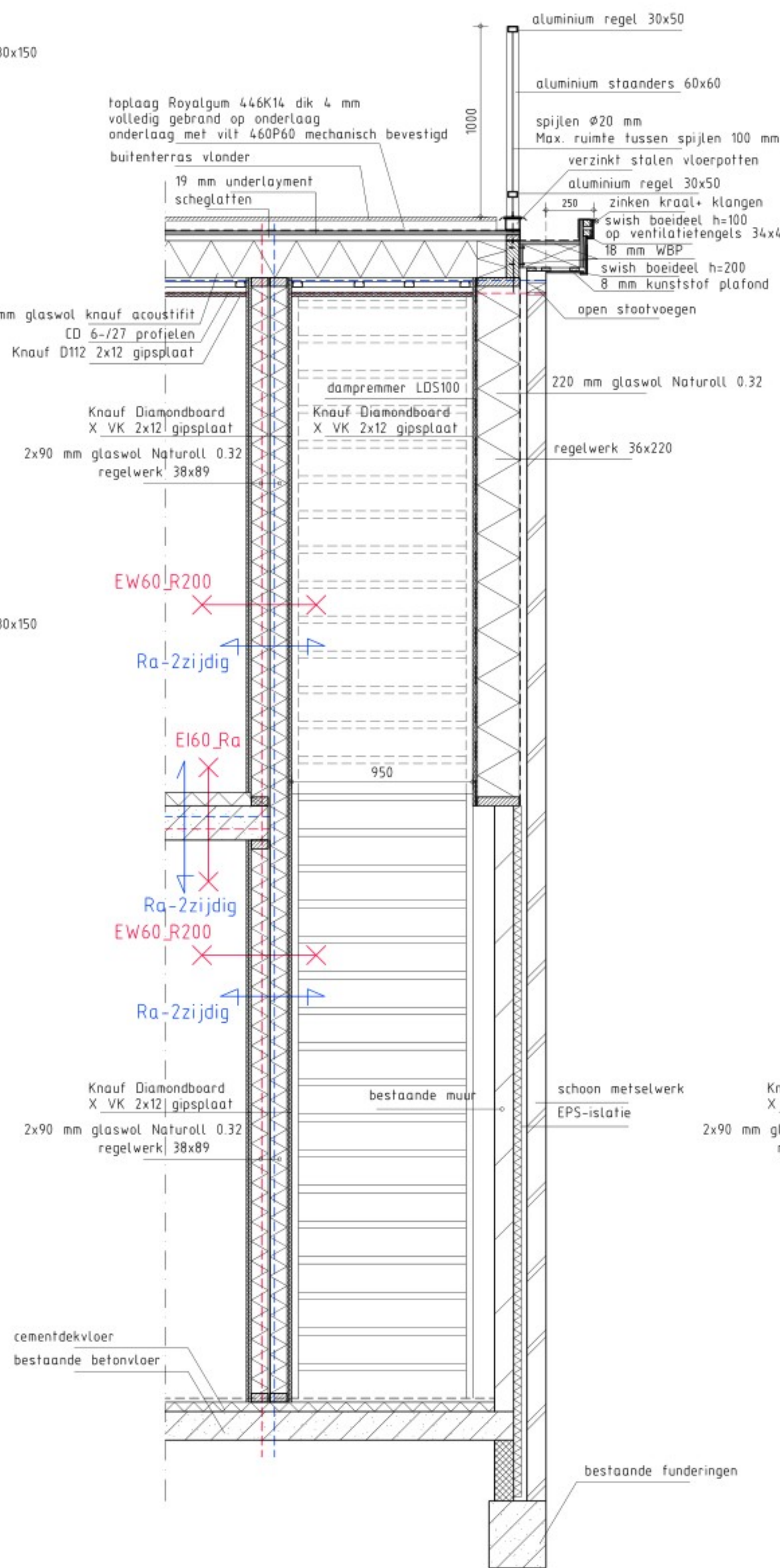
Doorsnede D
