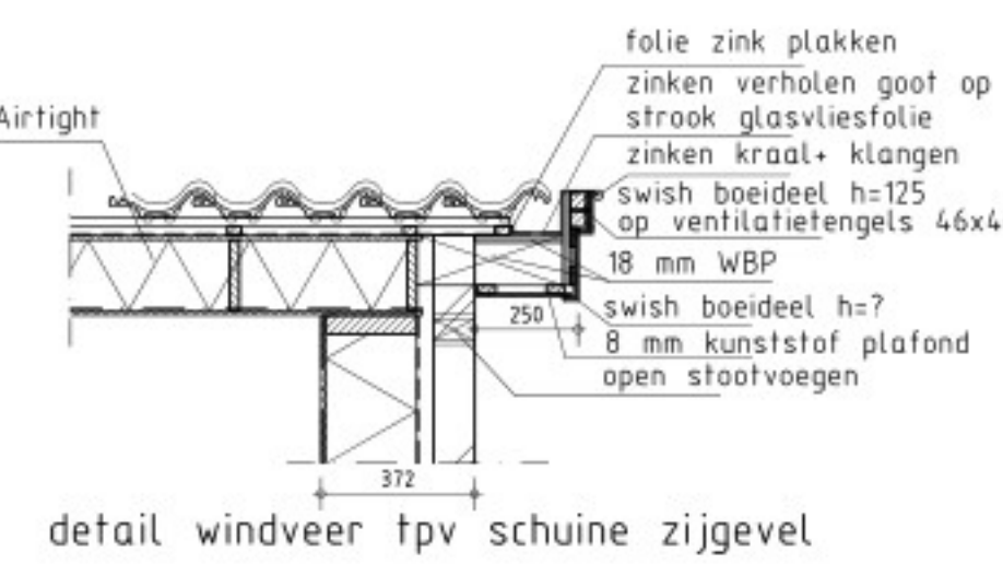
detail windveer tpv schuine zijgevel
