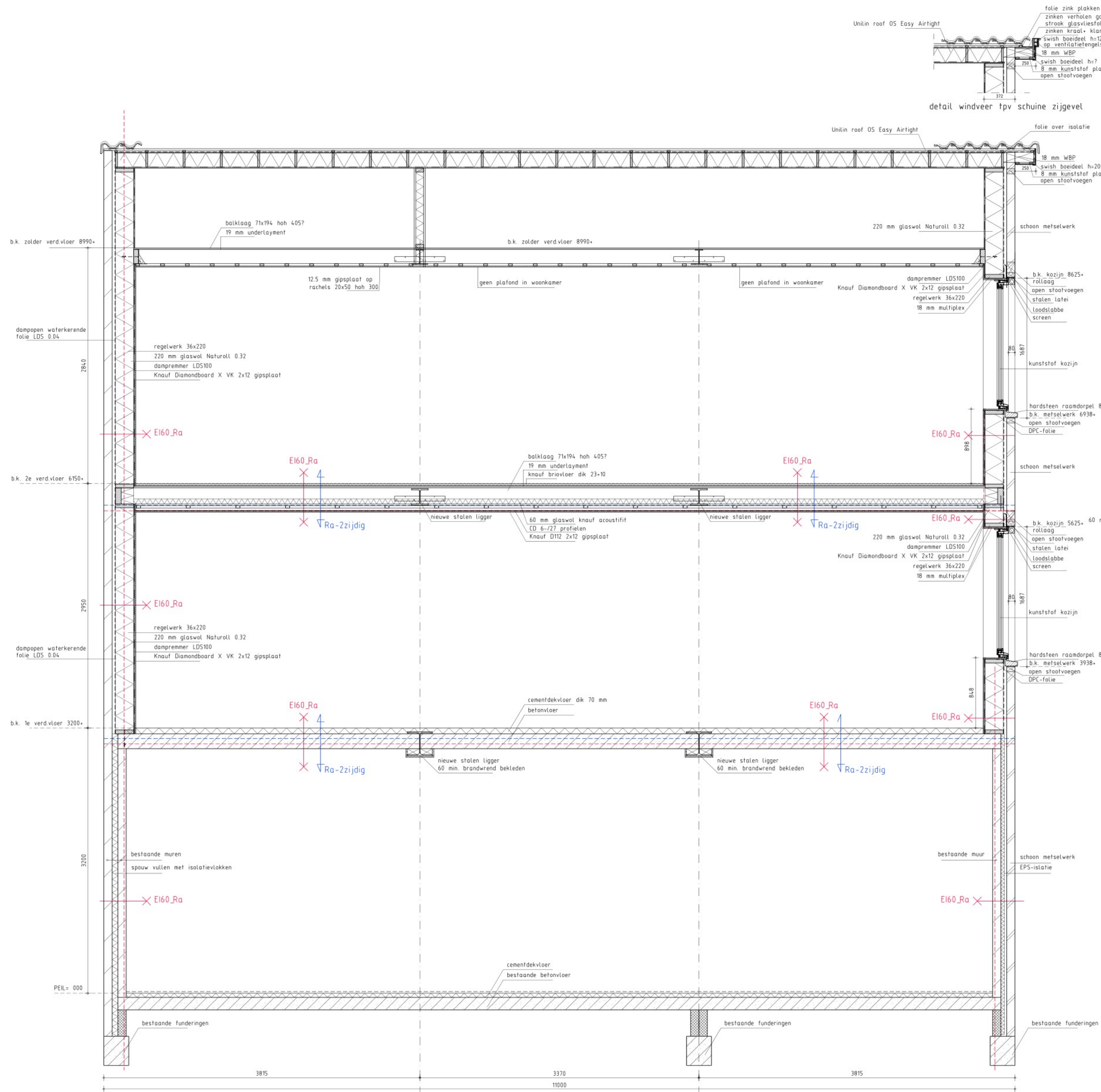
Doorsnede C-C
