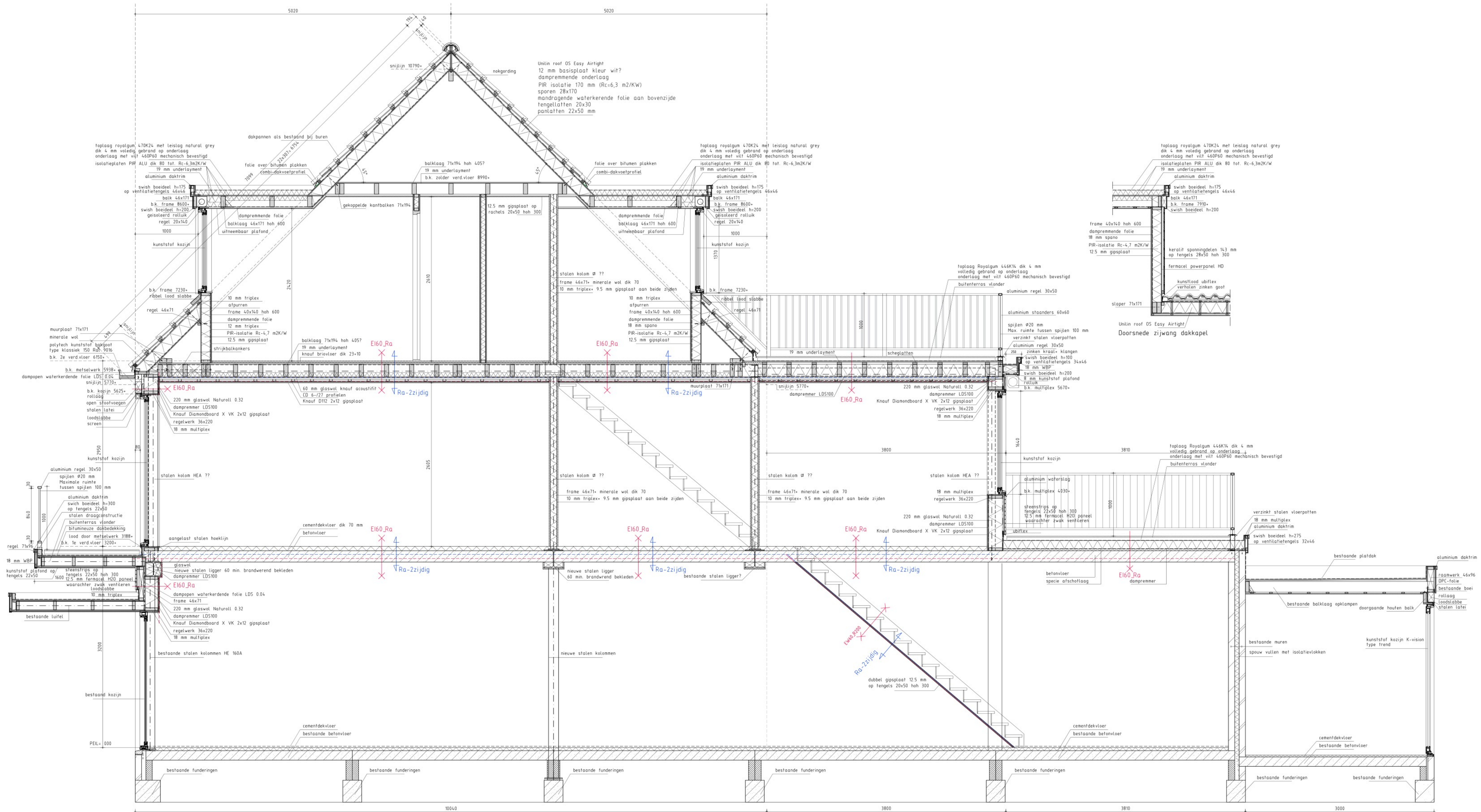
Doorsnede A-A
